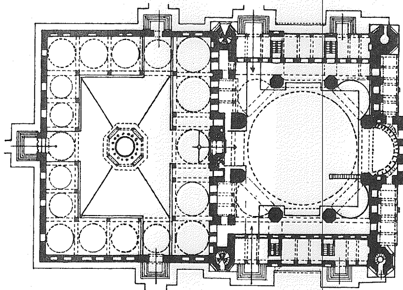
Εικ. 84. Σελιμιέ Τζαμί, κάτοψις.
